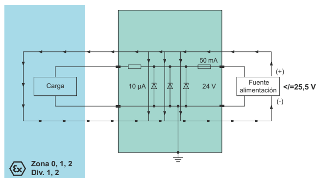
Figura 5 Corriente de fuga a través de los diodos zener
