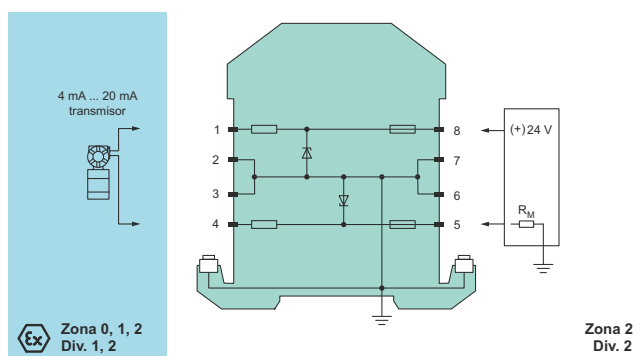
Figura 13 Barrera Zener de dos canales
