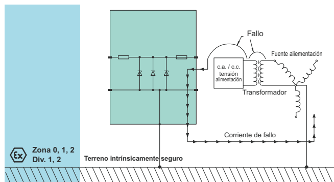
Figura 8 Barrera Zener con puesta a tierra
