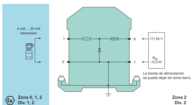
Figura 12 Barrera Zener de un solo canal
