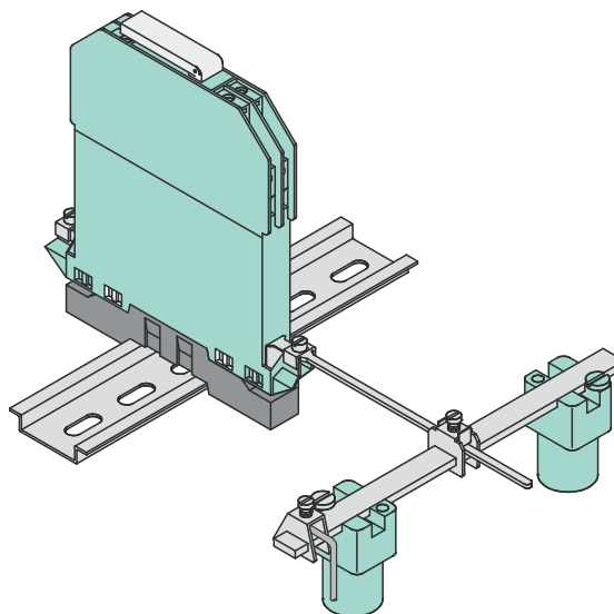
Figura 11 Montaje aislado (puesta a tierra individual)
