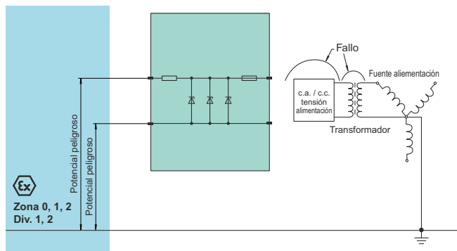
Figura 7 Barrera Zener sin puesta a tierra
