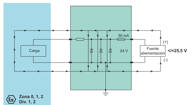
Figura 6 Drenaje de corriente total de los diodos zener
