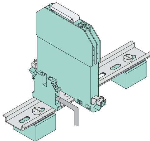
Figura 10 Montaje aislado (puesta a tierra por grupo)
