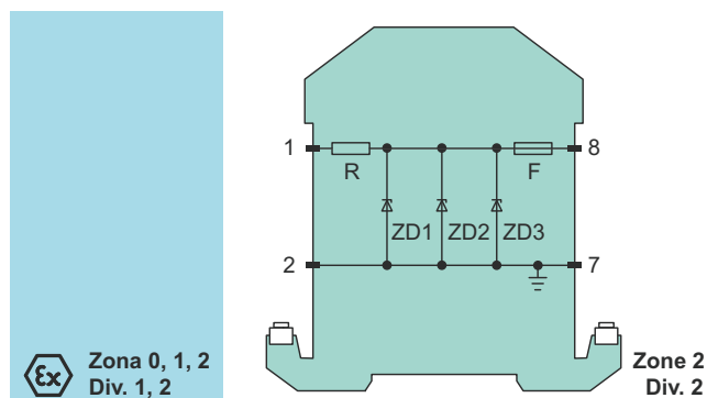
Figura 4 Diagrama del circuito
