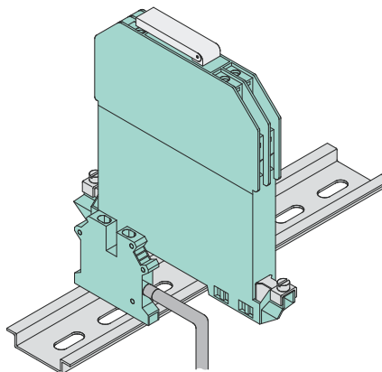
Figura 9 Conexión equipotencial a través del carril din
